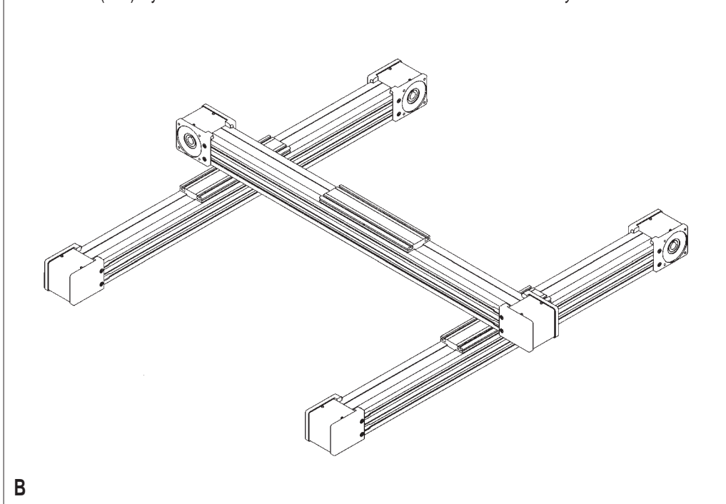
Zwei-Achsen (X-Y)-System
